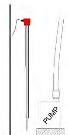
Bild 16: Nivågivare och vattenpump i pumpbrunn
